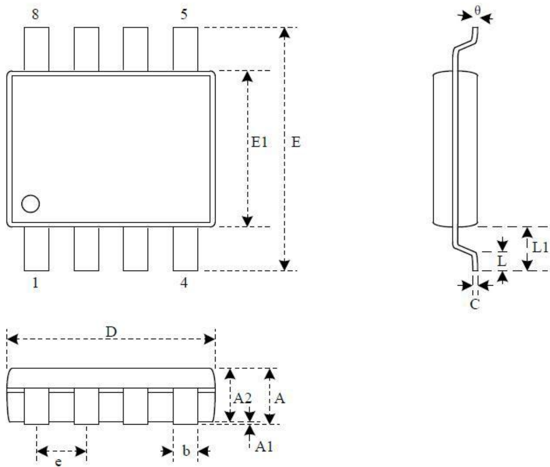
Dimensions
