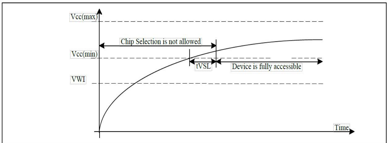
上电时序
